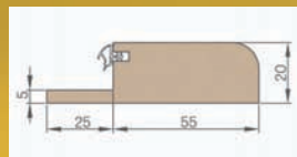
Próg z twardego drewna liściastego szer. 55 mm, lakierowany bezbarwny
