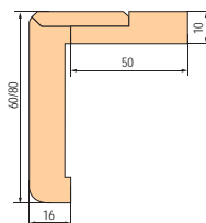
Opaska kątowa 60/80 mm z klipsem MDF za dopłatą
