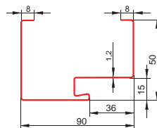
Ościeznica stalowa z uszczelką FD-25/21B
