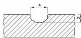
Schemat aplikacji frezowanej
